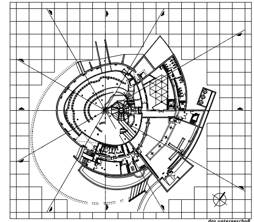
das untergeschoß
